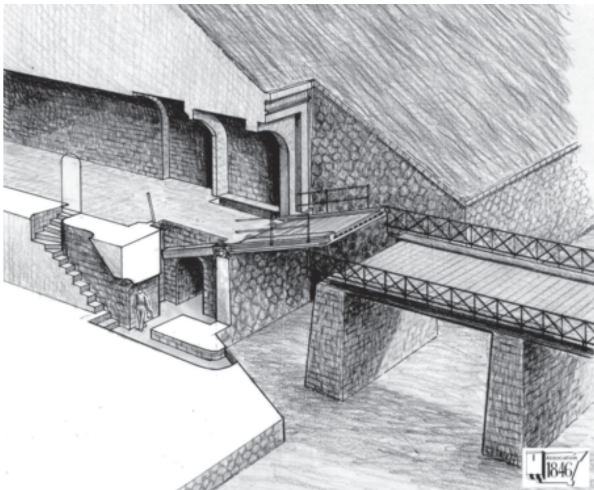
Fig. 5. – Vue en écorché de la porte du réduit et du système du pont-levis. Dessin Lionel Duigou.
