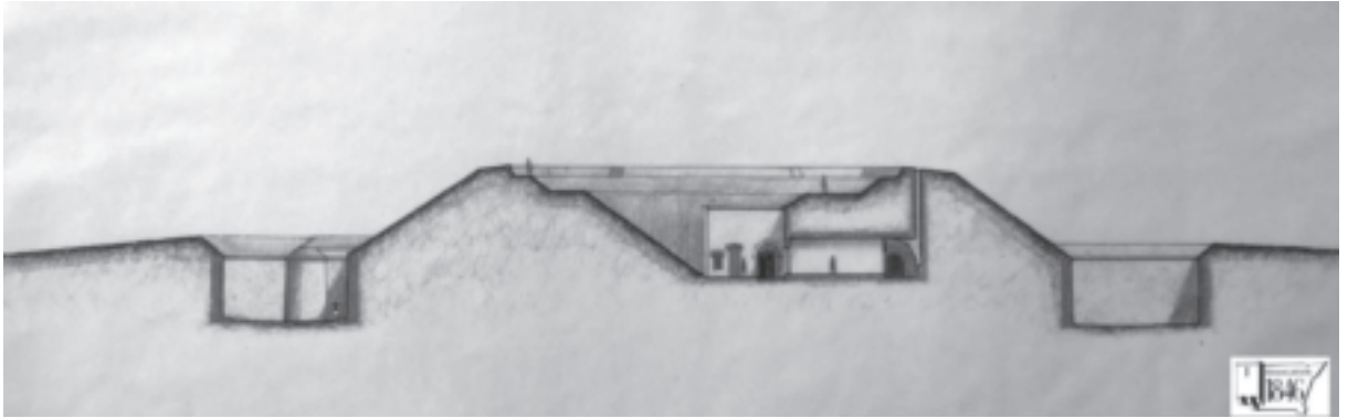
Fig. 2. – Coupe du réduit au niveau d'une des cours. Le casernement voûté tourne le dos à l'ennemi. Dessin Lionel Duigou.
