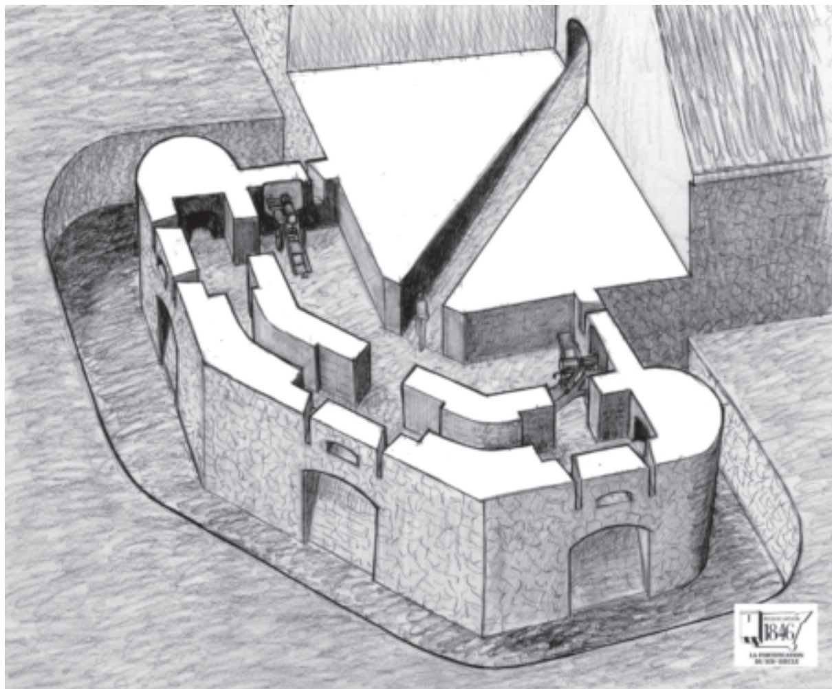
Fig. 4. – Vue en écorché de la caponnière double. Dessin Lionel Duigou.
