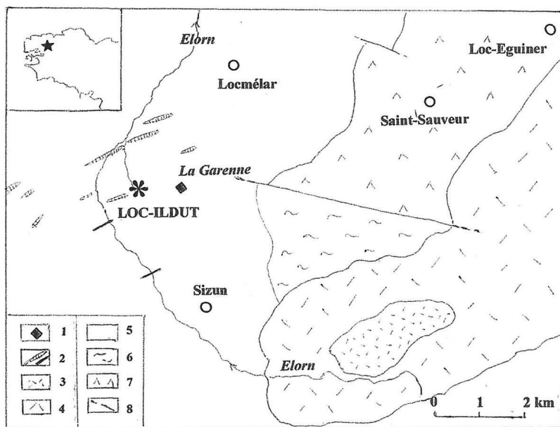
Fig. 19. – Esquisse géologique des environs de Loc-Ildut. D'après les cartes géologiques au 1/50 000 « Le Faou » (1982) et « Landerneau » (2010), éd. BRGM. Pour le secteur examiné, levés de L. Chauris, J.-R. Darboux, J. Garreau et B. Hallégouët. 1. Grès ferrugineux pliocène. 2. Filons de microgranite et de kersanton (trait noir). – 3 et 4. Massif granitique de Plounéour-Ménez (3 : faciès à grain fin ; 4 : faciès à gros grain). 5. Paléozoïque (principalement Dévonien). – 6. Briovérien. 7. Orthogneiss. – 8. Faille.
