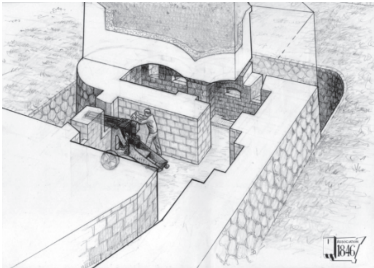
Fig. 3. – Vue en écorché d'une des caponnières simples avec son canon-revolver en action. Dessin Lionel Duigou.
