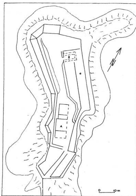
Fig. 2. – Plan schématisé du fort de Blosson.
