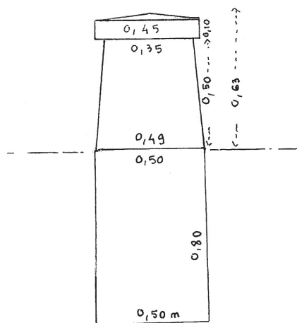
Fig. 3. - Élévation d'une borne pour le môle projeté à Pempoul.
