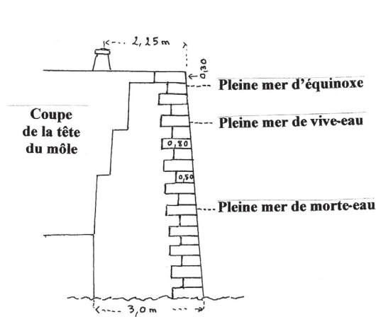
Fig. 2. - Coupe de la tête du môle projeté à Pempoul.
