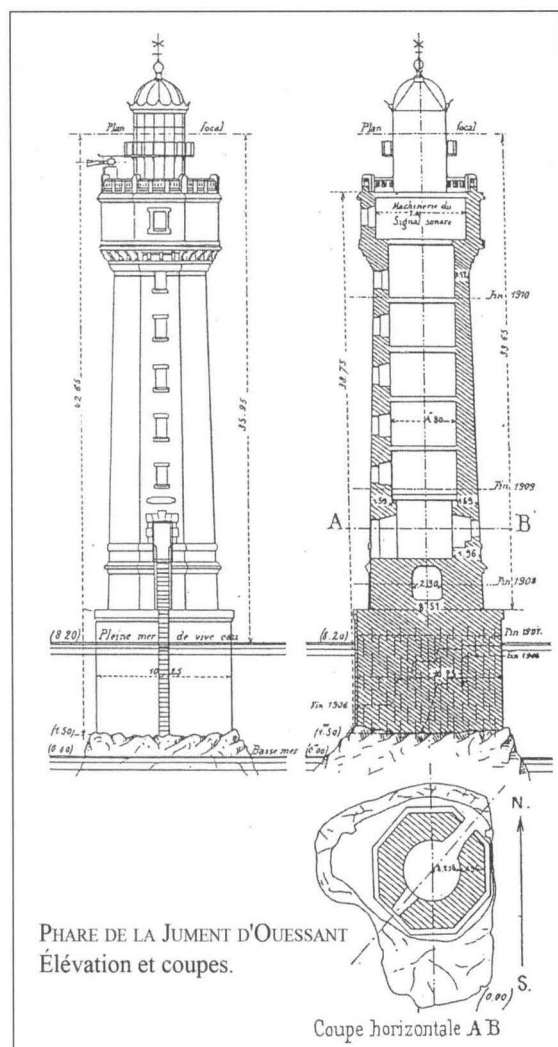
Fig. 12. – Phare de la Jument.
