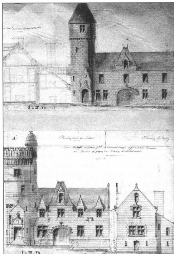
Fig. 5. – Projets de l'aile occidentale, s.d. Arch. dioc. Quimper, 8 L IV 53, 54.
