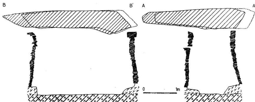
Fig. 5. — Coupes longitudinale et transversale du caveau.
