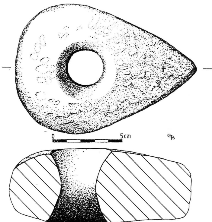
Fig. 9. — Saint-Coulitz, dessin de la hache-marteau de Penhoat . Dessin : B. Grall.
