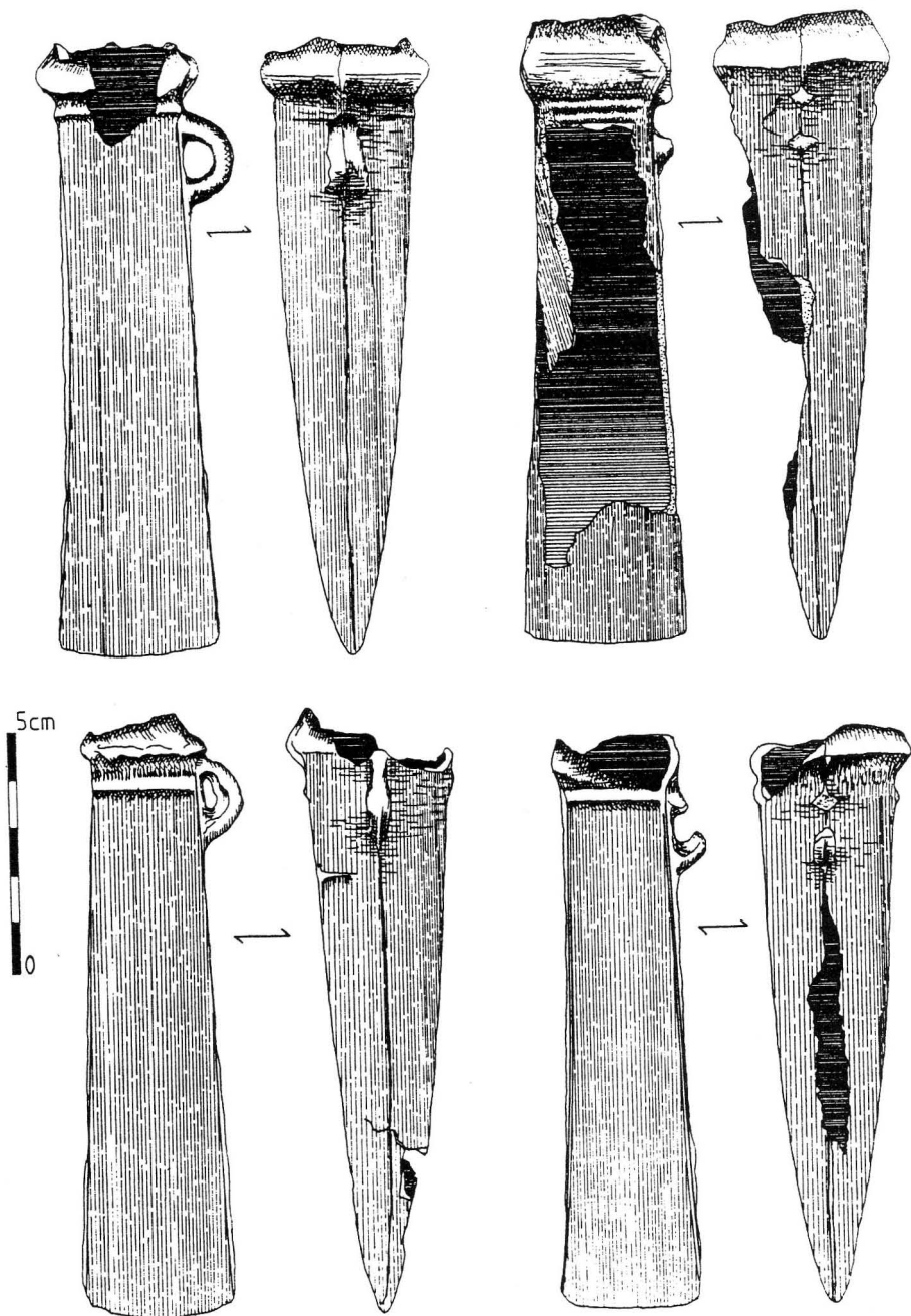
Fig. 12. — Landrévarzec, dessin de quatre des douze haches à douille découvertes à Kervouelet.
