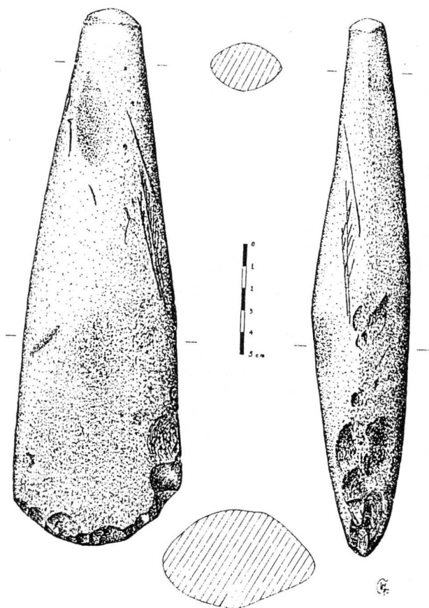
Fig. 7. — Guerlesquin, dessin de la hache à bouton en dolérite provenant d' Ar-Goarem .
