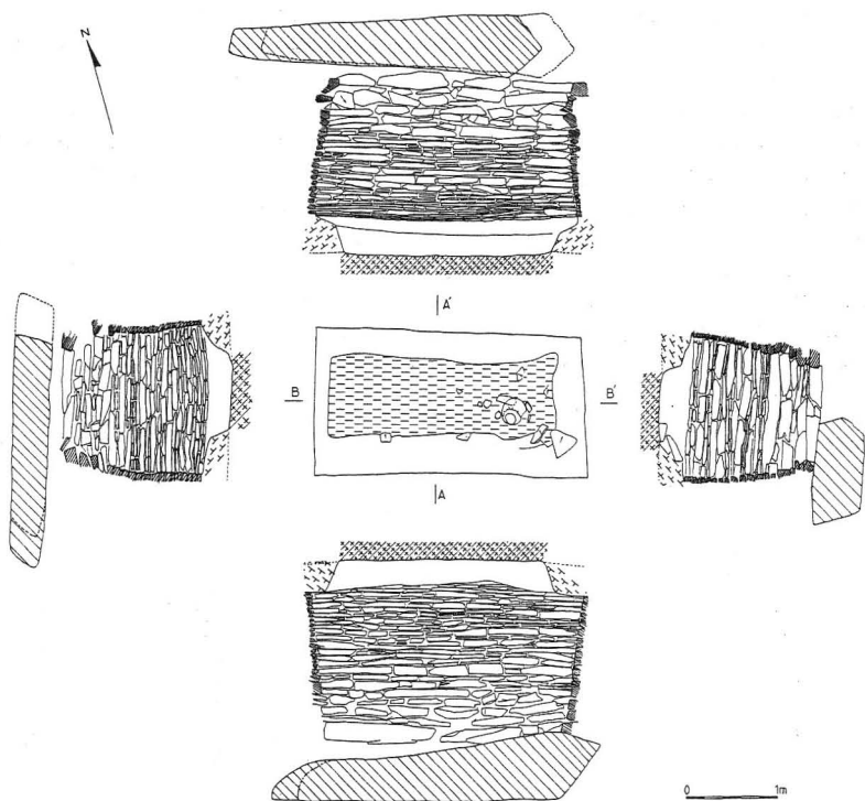
Fig. 4. — Plan du caveau et élévations internes des parois. La position originelle de la dalle est figurée en pointillé.
