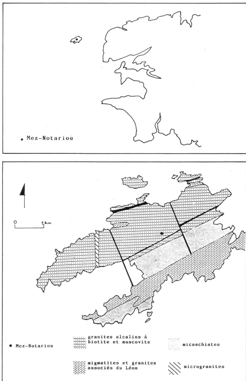
Fig. 1. — Localisation et géologie d'Ouessant.
