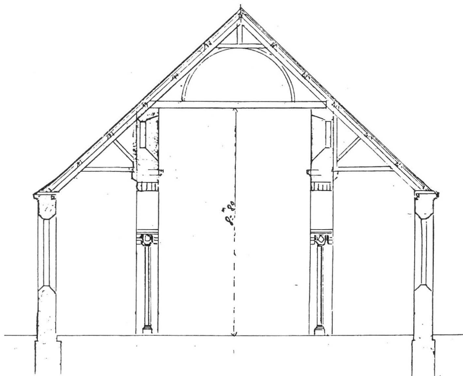
Fig. 3. — Ancienne église de Scaër, croquis de Joseph Bigot.
