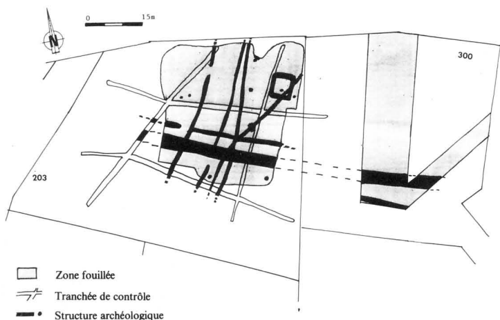
Fig. 11. — Quimper, Kernénez, ensemble des vestiges des parcelles 203-300.
