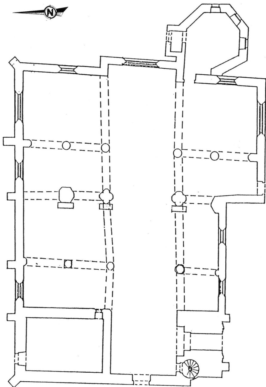
Fig. 5. — Plan de la chapelle Sainte-Marie du Ménez-Hom.
