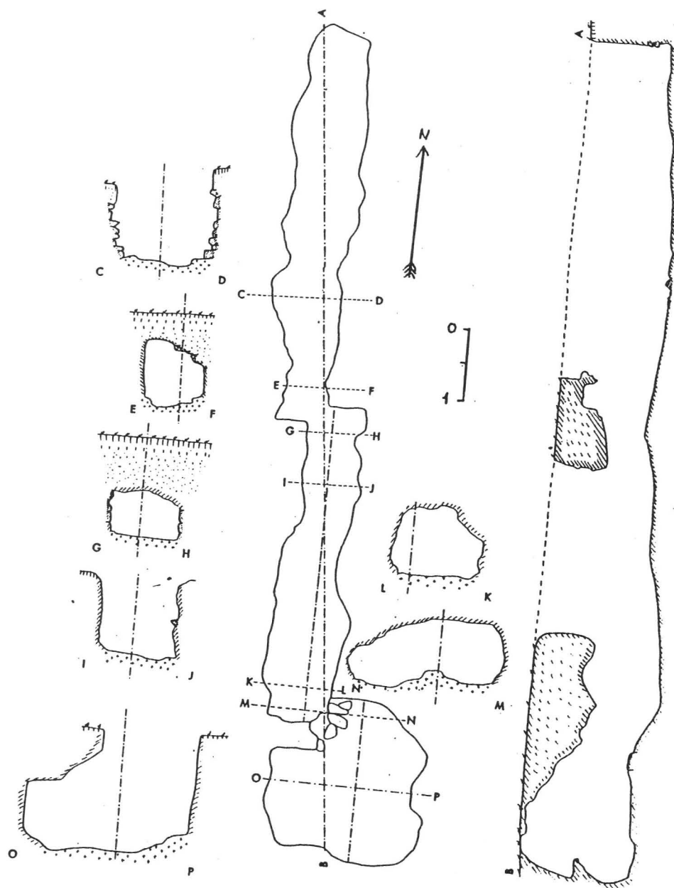
Fig. 2. — Plan et sections du souterrain. Plan au fond; pour le contour de surface, se reporter au plan d'ensemble.
