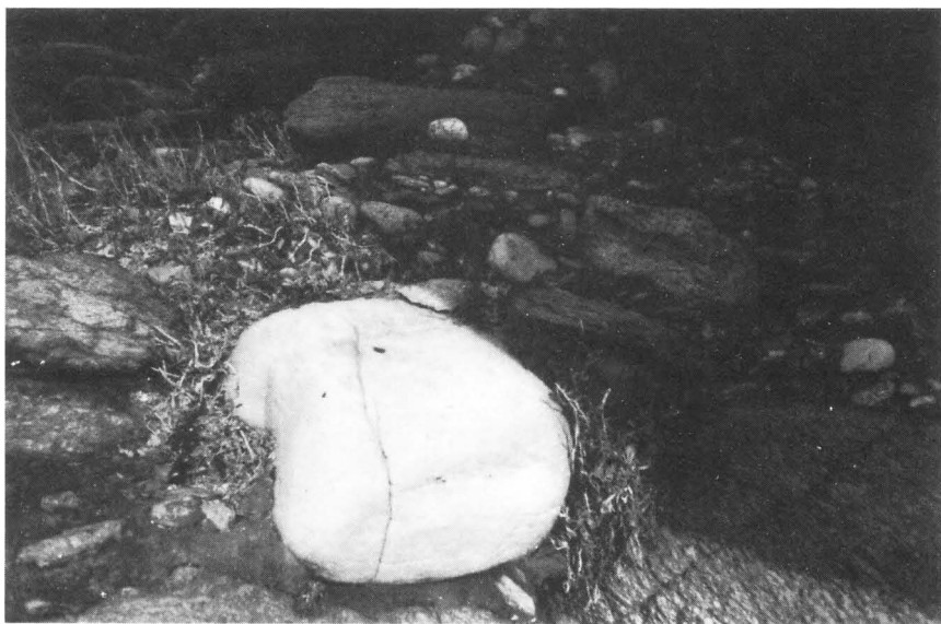
Fig. 3. — Porsliogan, galets anciens cimentés par l'oxyde de fer.
