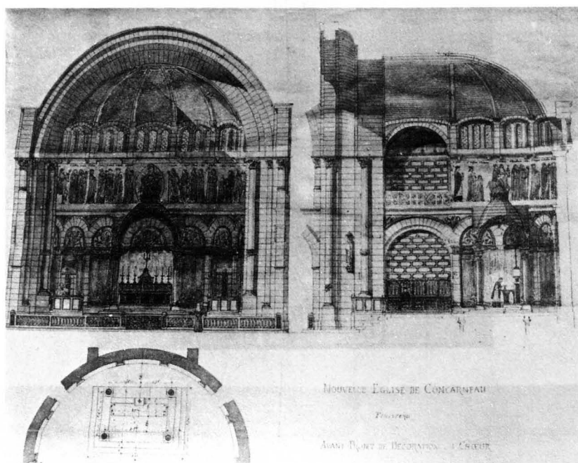
Fig. 4. — Coupe de la nouvelle église.
