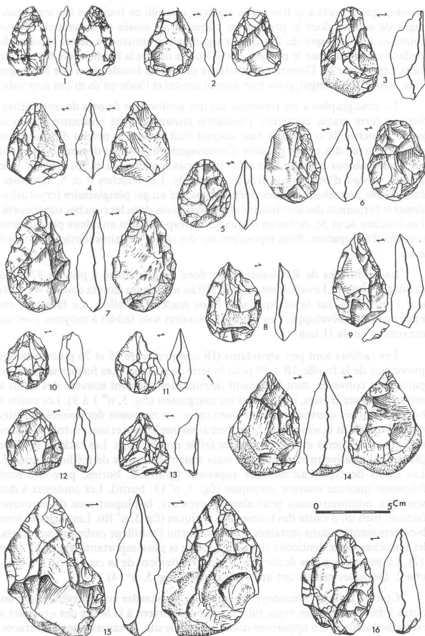
Fig. 3. — Kerlouan, Tréissény , bifaces (dessins de Y. Onnée).
