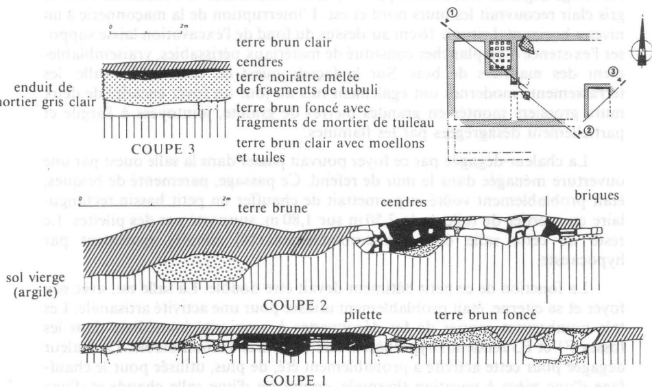
Fig. 4. — Plan et coupe des thermes.
