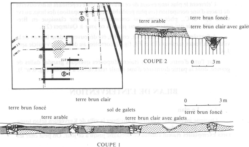
Fig. 5. — Coupes dans la villa.
