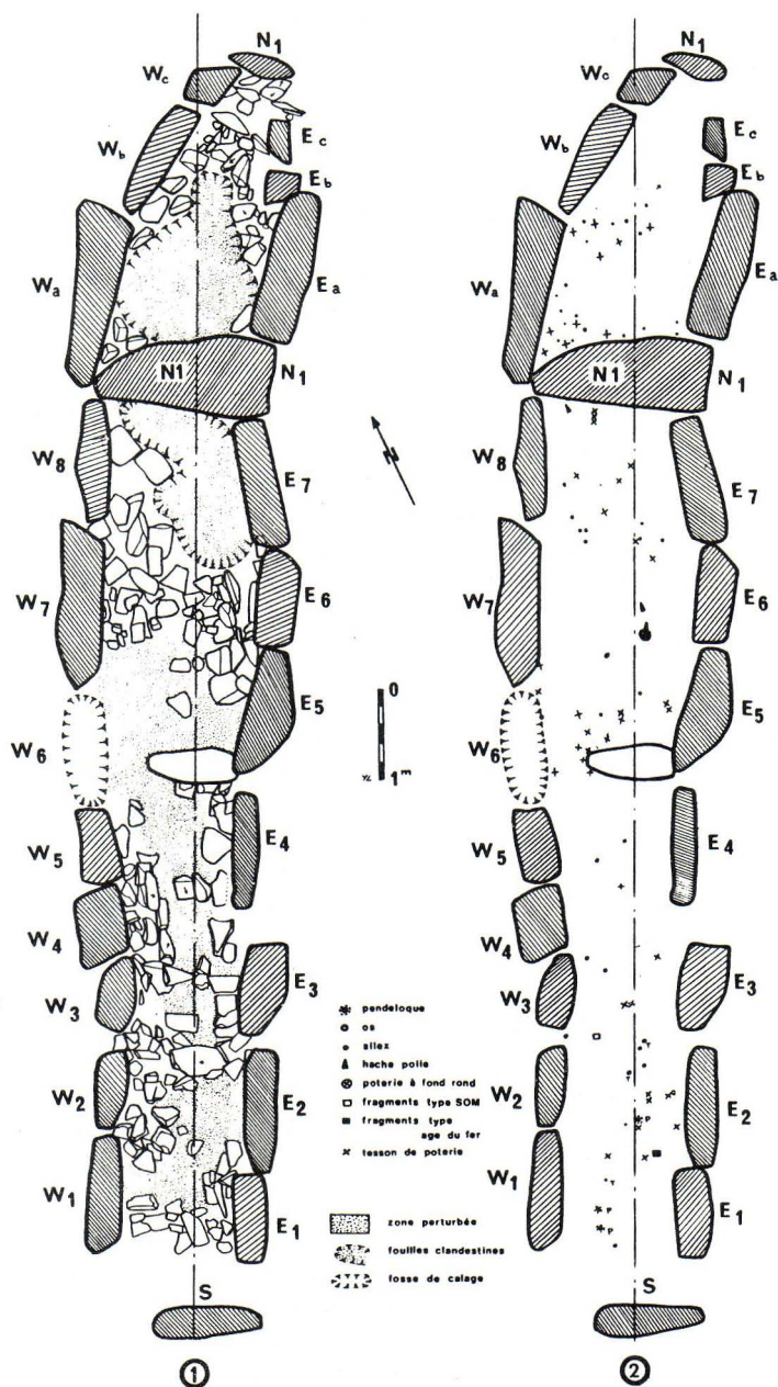
Fig. 2. — Plouescat, Kernic, l'allée couverte.
