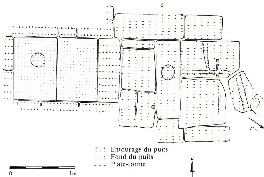
Fig. 8. — Quimper, rue Saint-Valentin , plan général de la fontaine.
