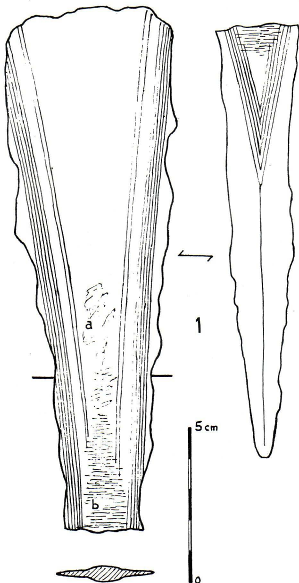
Planche I. — Saint-Nic, dépôt de Kermot . N° 1: Épée, masse: 210 g, dimensions: 312 × 58 × 5 mm a: traces anciennes d'enlèvement de métal b: microfissures anciennes dues au pliage
