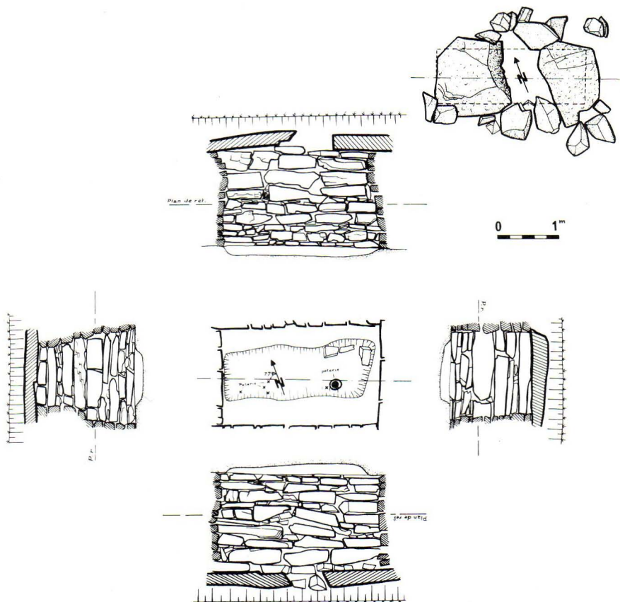
Fig. 4. — Plouigneau, caveau funéraire de La Chapelle du Mur . Plan de la tombe.
