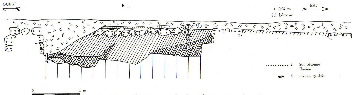
Fig. 10. — Saint-Evarzec, Le Cavardy , coupe stratigraphique. Selon 10-11.
