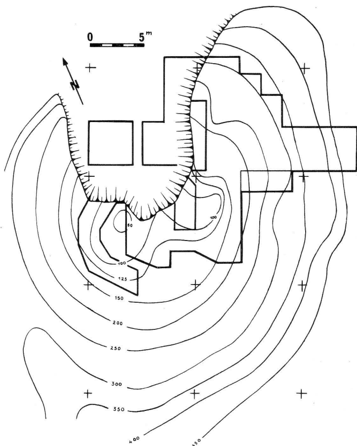
Fig. 2. — Saint-Thois, cairn de Ty-Floc'h , plan masse. Contour de la carrière, courbes de niveau, implantation des fouilles.
