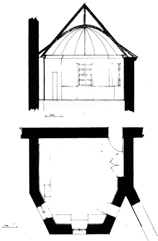
Fig. 1. — Brasparts, église Saint-Tujen, sacristie sud-est. Plan et coupe.
