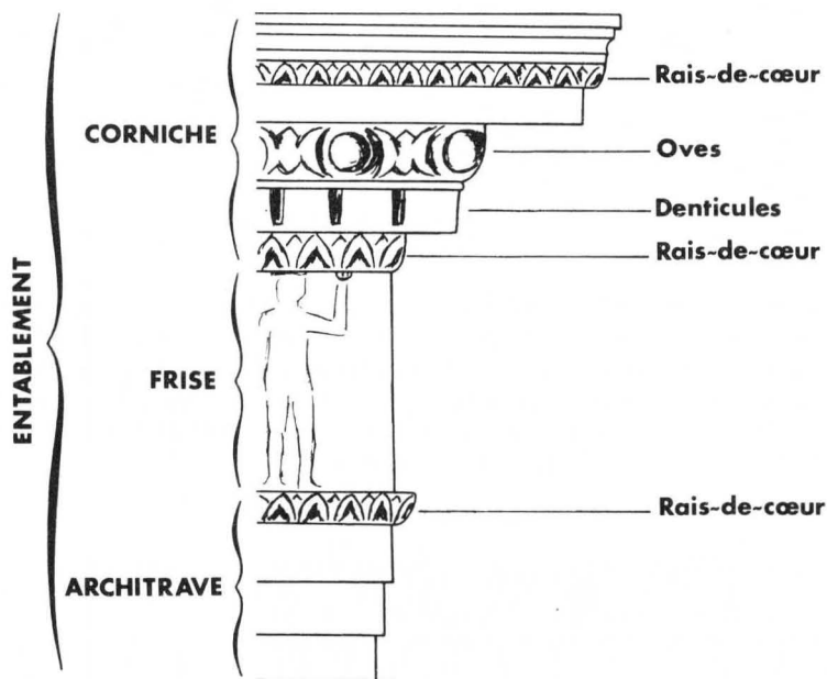
Fig. 2. - Exemple d'entablement dans l'ordre ionique.
