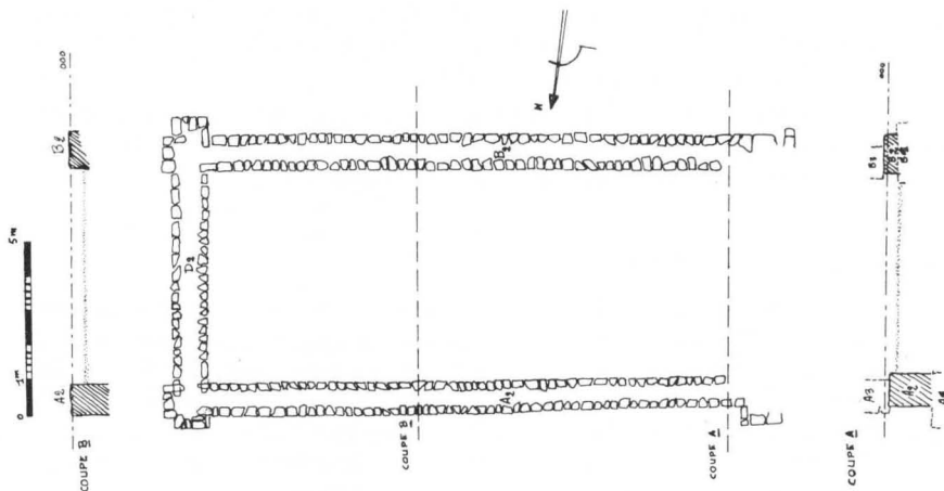
Fig. 5. - Plan de la chapelle II.
