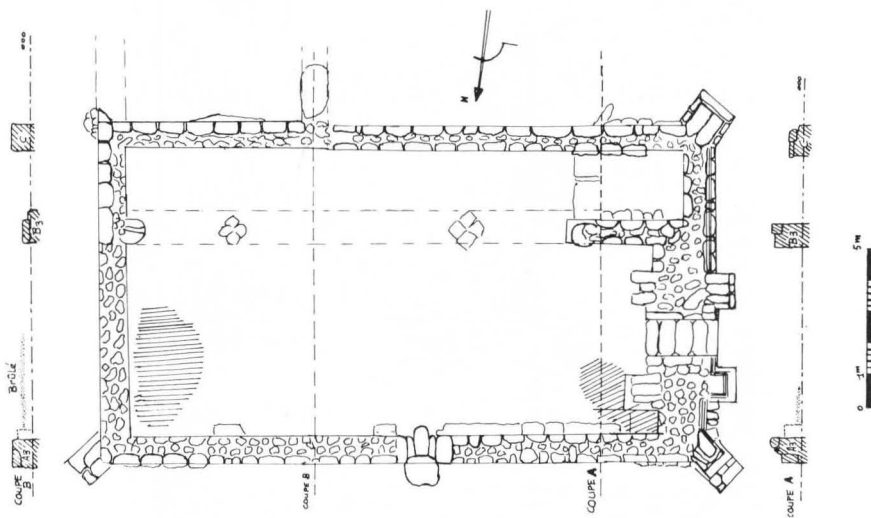
Fig. 3. - Plan de la chapelle III.
