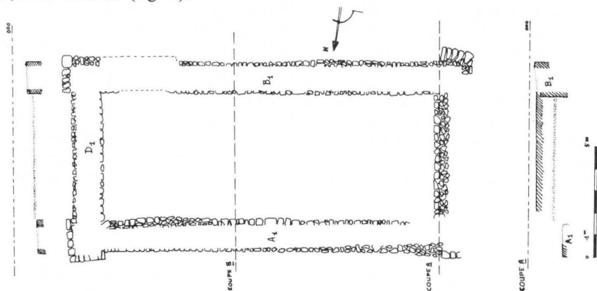
Fig. 7. - Plan de la chapelle I.
