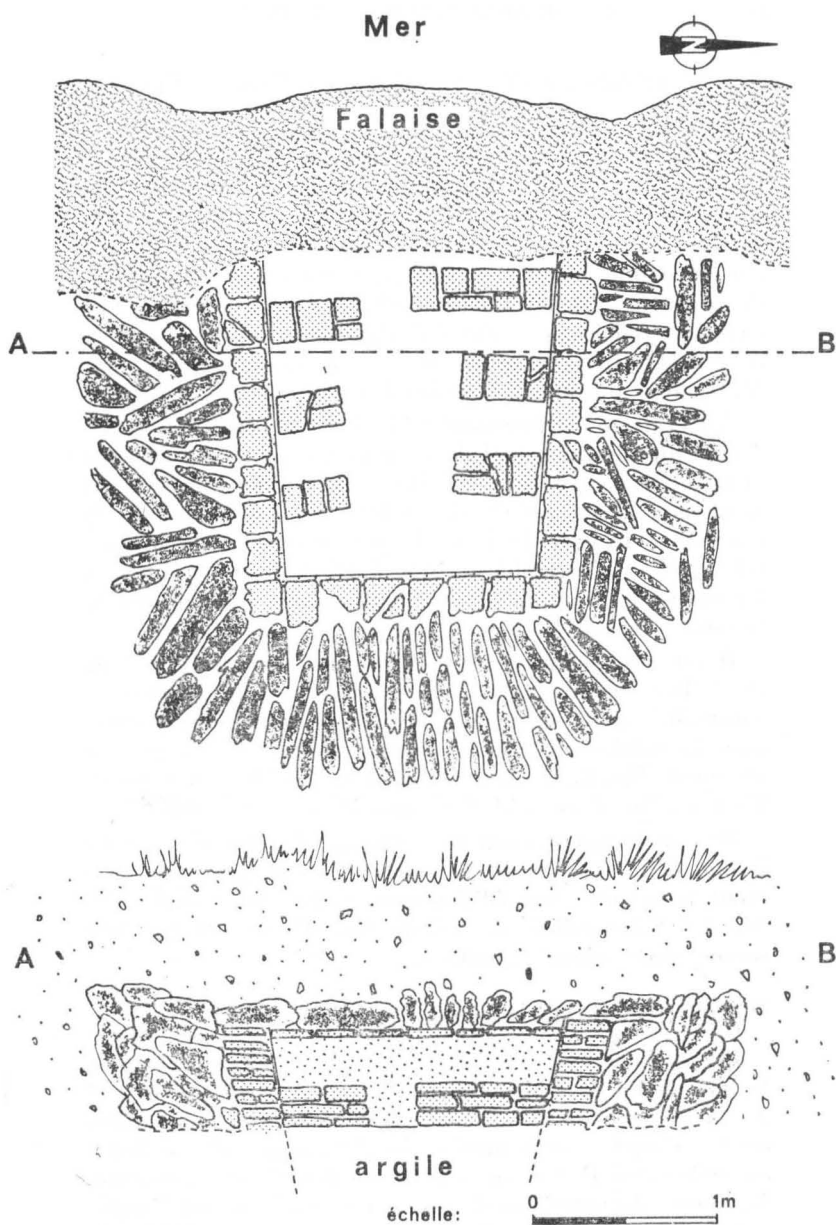
Fig. 7. — Plan du four de Sainte-Anne-La-Palud, en Plo-névez-Porzay.
