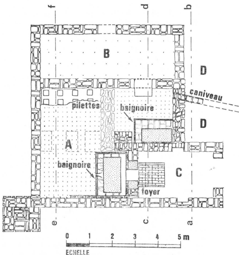
Fig. 4. — Plan des bains du Valy-Cloistre, en La Roche-Maurice.
