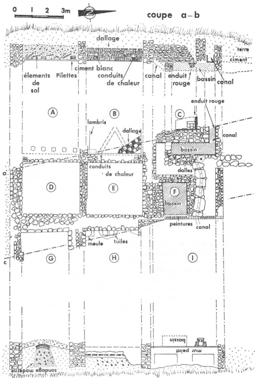
Fig. 8. — Villa gallo-romaine de Kervénennec, en Pont-Croix (plan et coupe au 1-4-71).
