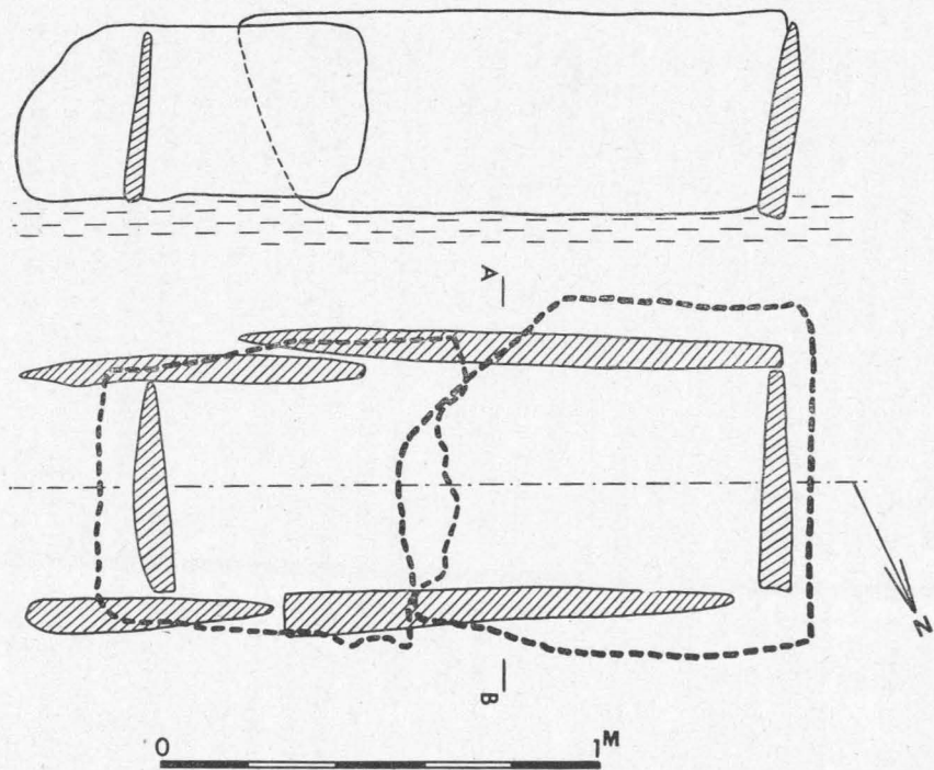
Plan, élévation latérale et coupe du coffre de Menez- Banal, en Landeleau (relevé par J. Briard).
