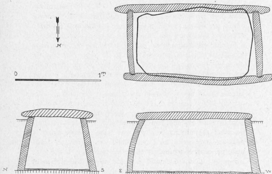
FIG. 2. — COFFRE DE L'ANSE BERTHEAUME, EN PLOUGONVELIN Plan du coffre et sections
