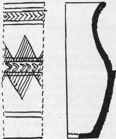
FIG. 3. — Reconstitution du profil du vase de Maez bihan à Kergoz, en Plounévez-Lochrist (1/3).
