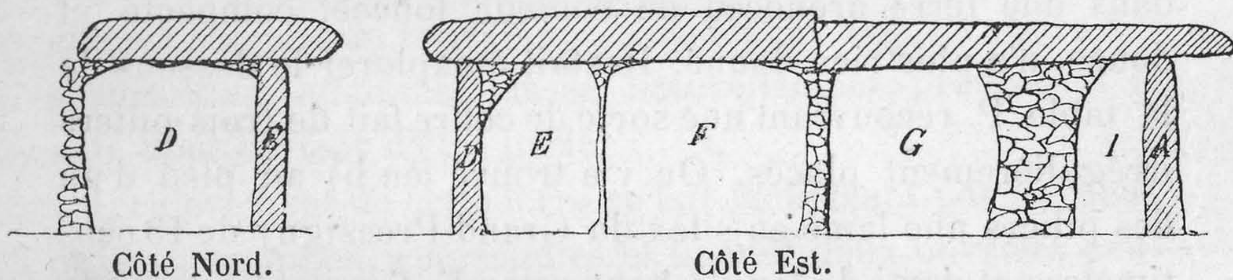
ÉLEVATION DES COTÉS DE LA CHAMBRE NORD (1/100).
