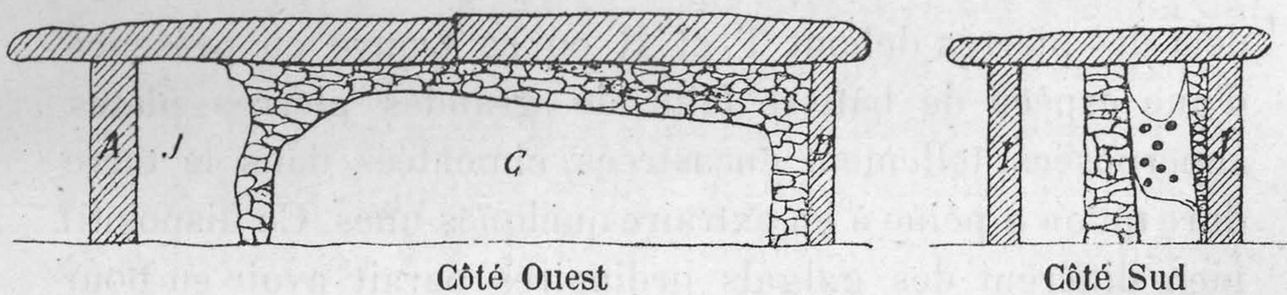
ÉLEVATION DE DEUX DES COTÉS DE LA CHAMBRE NORD (1/100)
