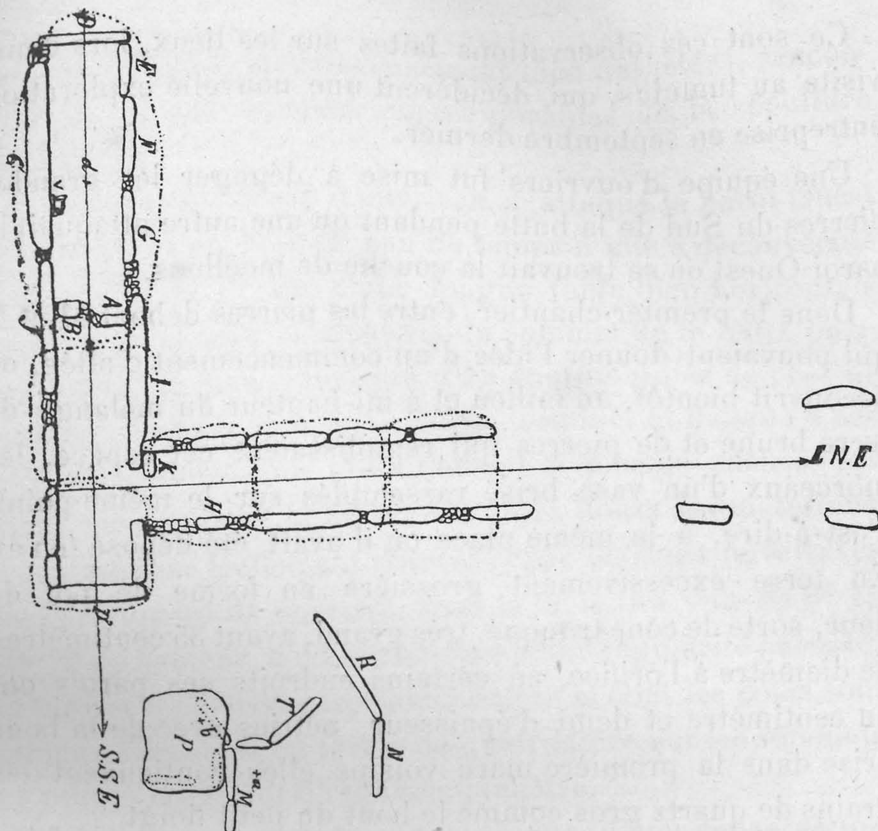
PLAN (1/200).
